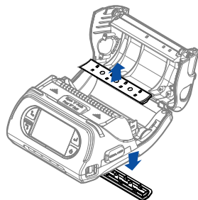
외장용지 덮개
